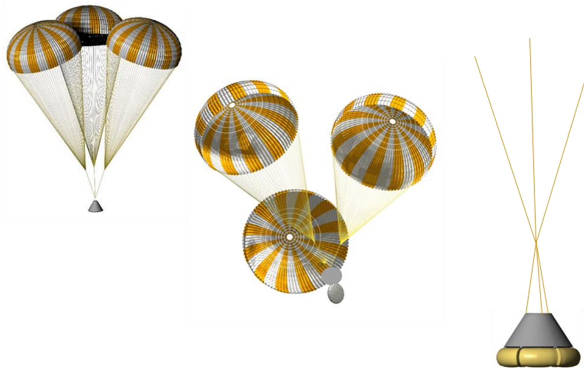
Figure 7: ALS Operational Sequence
